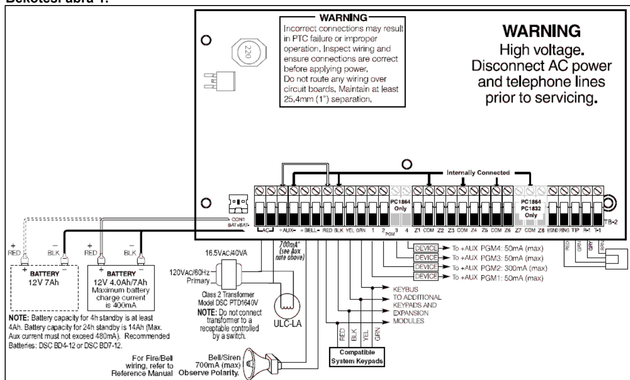
Bekötési ábra 1.
