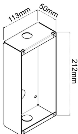
2 modulós süllyesztődoboz
