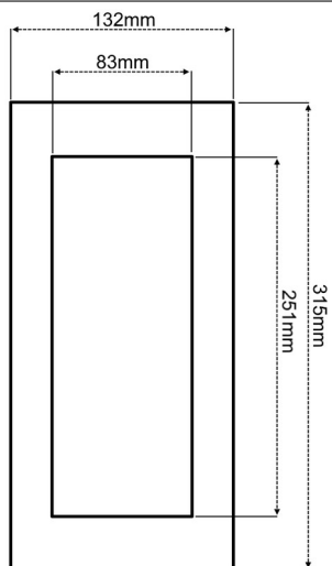
2 modulós süllyesztődoboz
