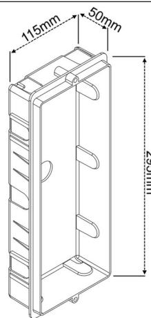
3 modulós süllyesztődoboz
