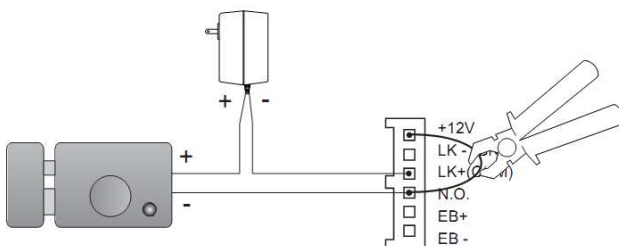
Normál üzemmódú zár bekötése külső táp használatával
