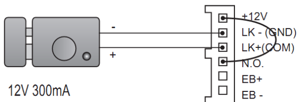
Normál üzemmódú zár bekötése
