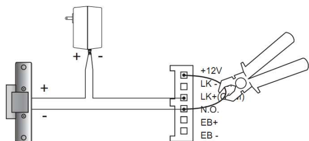
Fordított üzemmódú zár bekötése külső táp használatával
