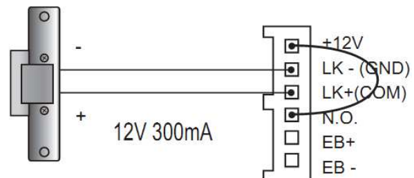
Fordított üzemmódú zár bekötése
