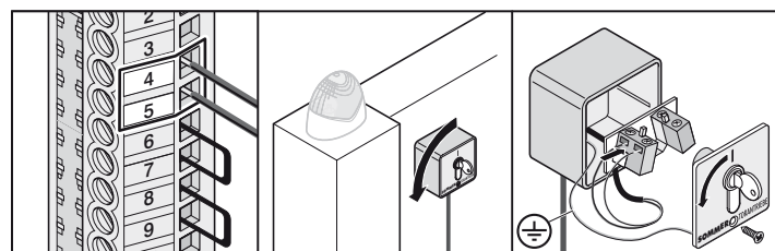
2. nyomógomb 4 + 5 kapocs
