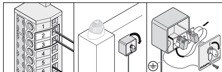
1. nyomógomb 2 + 3 kapocs
